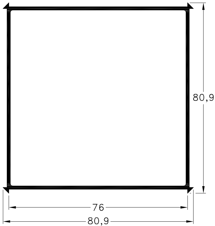
1010455 - Columna Acople a 90° / 180° Peso: 1,18 Kg/m. Largo Std.: 6.030 mm.
