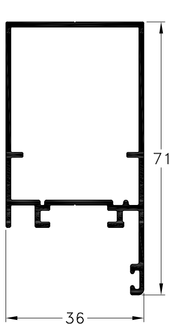
1032981 - Parante Peso: 0,79 Kg/m. Largo Std.: 6.200 mm.
