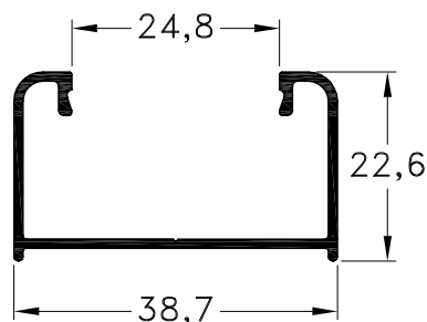
1032985 - Adaptador D.V.H. Peso: 0,30 Kg/m. Largo Std.: 6.030 mm.
