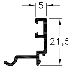
1020644 - Contravidrio Recto 5 mm. Peso: 0,18 Kg/m. Largo Std.: 6.030 mm.
