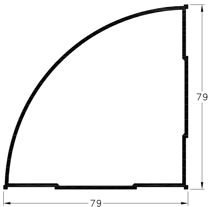
1010986 - Columna Curva Peso: 1,06 Kg/m. Largo Std.: 6.030 mm.
