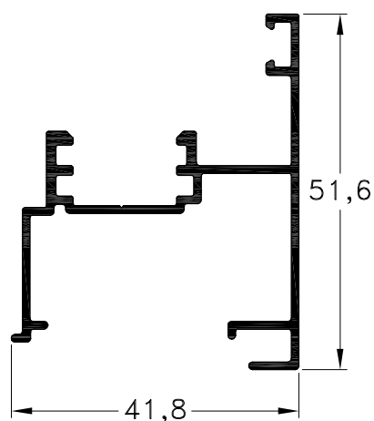
1032980 - Encuentro Central Ventana y Puerta de Rebatir Peso: 0,54 Kg/m. Largo Std.: 6.030 mm.
