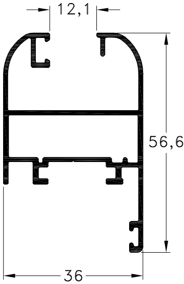
1032978 - Hoja V.S. Peso: 0,69 Kg/m. Largo Std.: 6.030 mm.
