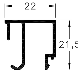
1020633 - Contravidrio Recto 22 mm. Peso: 0,26 Kg/m. Largo Std.: 6.030 mm.
