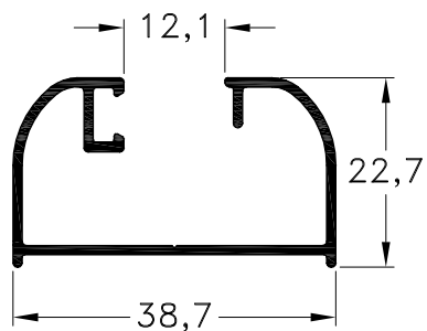
1032984 - Adaptador V.S. Peso: 0,35 Kg/m. Largo Std.: 6.030 mm.
