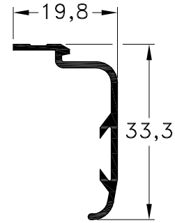
1010709 - Contramarco Peso: 0,19 Kg/m. Largo Std.: 6.150 mm.
