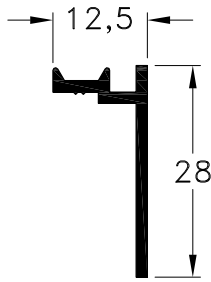
1010441 - Contramarco Peso: 0,18 Kg/m. Largo Std.: 6.150 mm.
