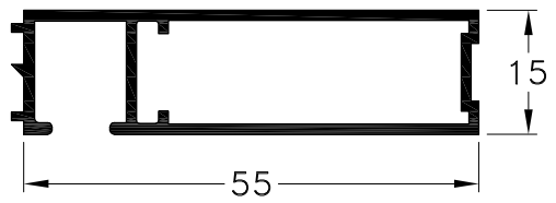
1010648 - Premarco de 55 mm. Peso: 0,50 Kg/m. Largo Std.: 6.150 mm.
