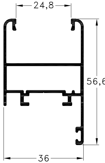
1032979 - Hoja D.V.H. Peso: 0,65 Kg/m. Largo Std.: 6.030 mm.
