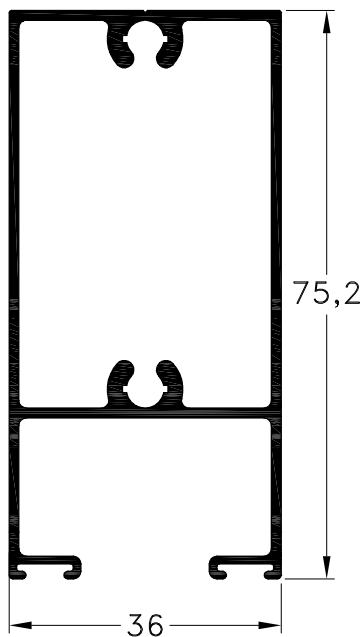
1032982 - Zócalo Peso: 1,01 Kg/m. Largo Std.: 6.030 mm.
