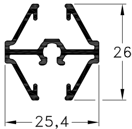
1010091 - Travesaño Vidrio Repartido Peso: 0,35 Kg/m. Largo Std.: 6.030 mm.
