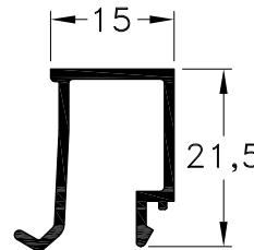
1020645 - Contravidrio Recto 15 mm. Peso: 0,21 Kg/m. Largo Std.: 6.030 mm.
