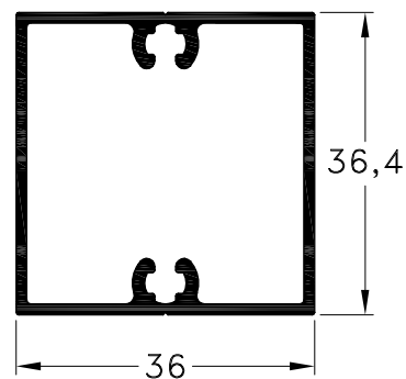
1032983 - Travesaño Peso: 0,61 Kg/m. Largo Std.: 6.030 mm.
