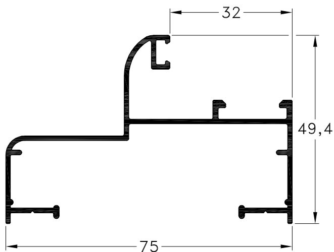
1032977 - Marco Peso: 0,72 Kg/m. Largo Std.: 6.200 mm.
