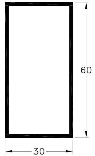
1090813 - Tubo 60 x 30 mm. Peso: 0,68 Kg/m. Largo Std.: 6.030 mm.
