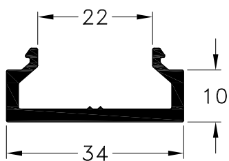
1090111 - Suplemento Zócalo Peso: 0,39 Kg/m. Largo Std.: 6.030 mm.
