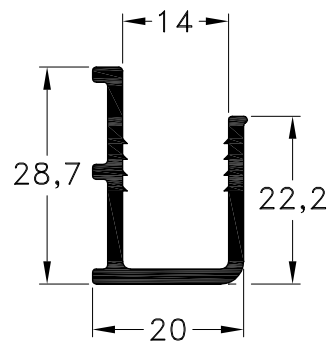
1090031 - Porta Blisan Inferior Peso: 0,38 Kg/m. Largo Std.: 6.030 mm.
