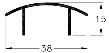
1090494 - Tapa Peso: 0,19 Kg/m. Largo Std.: 6.030 mm.
