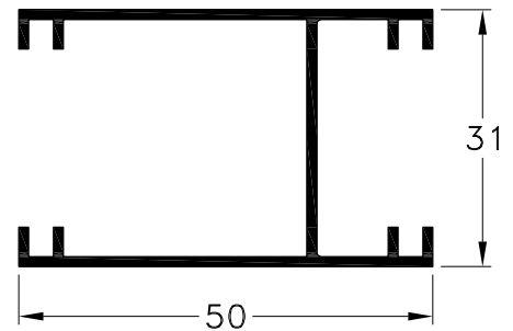
1090492 - Travesaño Peso: 0,54 Kg/m. Largo Std.: 6.030 mm.
