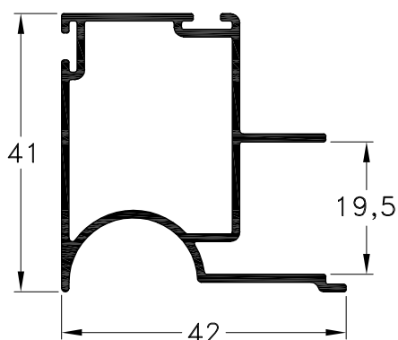
1090159 - Parante de 18 mm. Peso: 0,54 Kg/m. Largo Std.: 5.200 mm.
