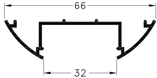
1090491 - Tapa Columna Peso: 0,40 Kg/m. Largo Std.: 6.030 mm.
