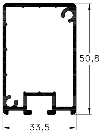
1090030 - Parante Peso: 0,83 Kg/m. Largo Std.: 6.030 mm.
