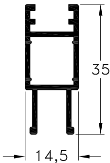
1090944 - Hoja Peso: 0,35 Kg/m. Largo Std.: 6.030 mm.
