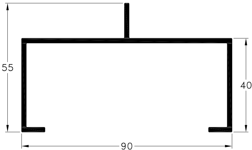
1090115 - Canal con Un Ala 90 x 40 mm. Peso: 1,06 Kg/m. Largo Std.: 6.030 mm.
