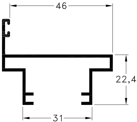
1090493 - Marco Peso: 0,48 Kg/m. Largo Std.: 6.030 mm.
