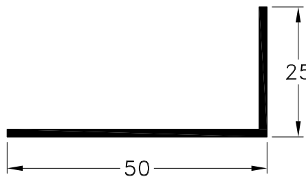
1090756 - Perfil Angulo Peso: 0,34 Kg/m. Largo Std.: 6.030 mm.
