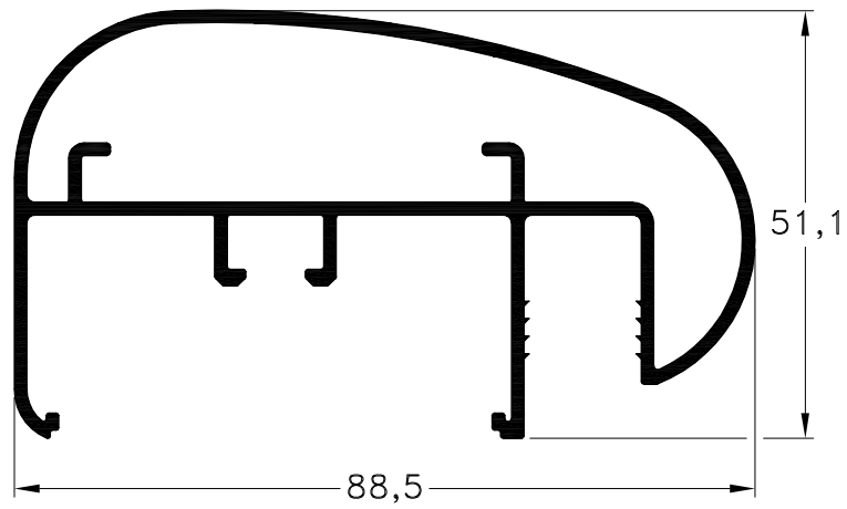
1090028 - Pasamanos Curvo Peso: 1,35 Kg/m. Largo Std.: 6.030 mm.
