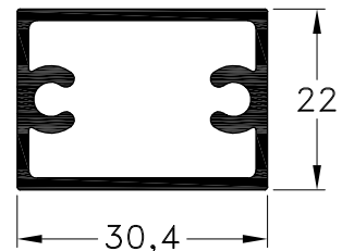
1090478 - Parante Angosto Peso: 0,51 Kg/m. Largo Std.: 6.030 mm.
