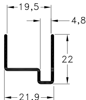
1090158 - Cantonera de 18 mm. Peso: 0,20 Kg/m. Largo Std.: 6.030 mm.
