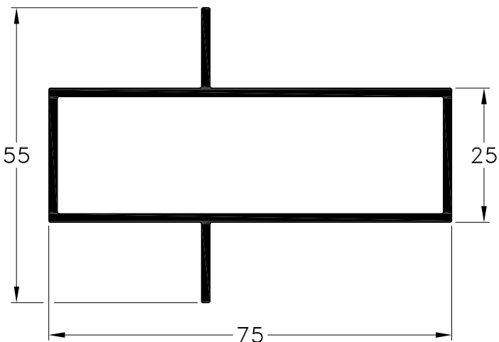
1090113 - Tubo con Dos Alas 75 x 25 mm. Peso: 0,97 Kg/m. Largo Std.: 6.030 mm.
