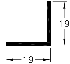
1090753 - Perfil Angulo Peso: 0,14 Kg/m. Largo Std.: 6.030 mm.
