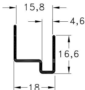
1090156 - Cantonera de 15 mm. Peso: 0,16 Kg/m. Largo Std.: 6.030 mm.
