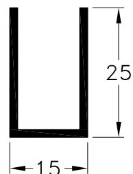
1090650 - "U" de Blindex Peso: 0,25 Kg/m. Largo Std.: 6.030 mm.
