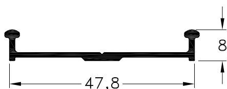
1090157 - Guía Inferior Peso: 0,25 Kg/m. Largo Std.: 6.030 mm.
