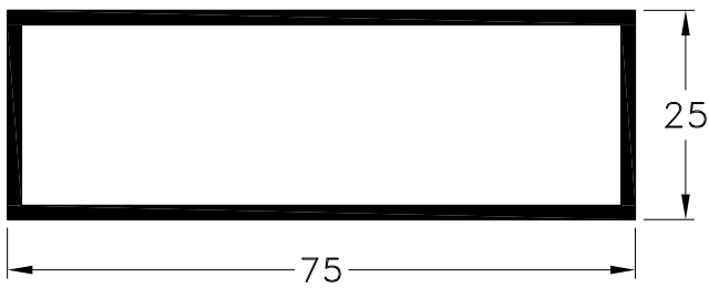
1090457 - Tubo 75 x 25 mm. Peso: 0,90 Kg/m. Largo Std.: 6.030 mm.
