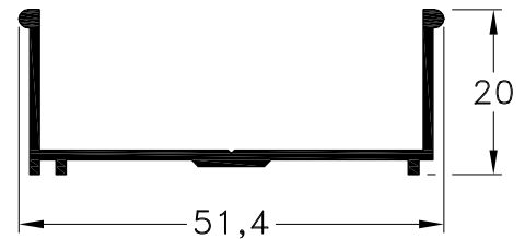
1090943 - Jamba Peso: 0,32 Kg/m. Largo Std.: 6.030 mm.
