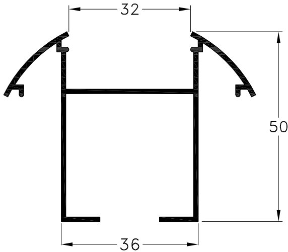
1090490 - Columna Peso: 0,67 Kg/m. Largo Std.: 6.030 mm.
