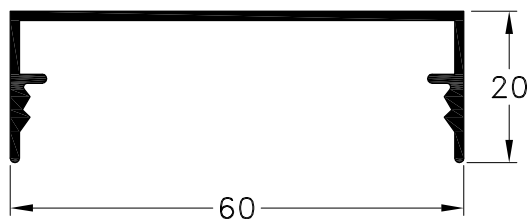
1080792 - Tapa Peso: 0,37 Kg/m. Largo Std.: 6.030 mm.
