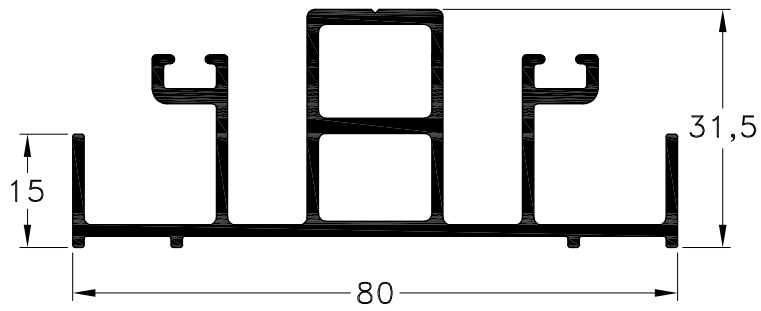
1090191 - Larguero Peso: 1,19 Kg/m. Largo Std.: 6.030 mm.
