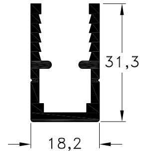
1090468 - Porta Vidrio Peso: 0,53 Kg/m. Largo Std.: 6.030 mm.
