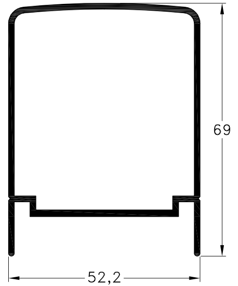
1090439 - Pasamanos Peso: 1,05 Kg/m. Largo Std.: 6.030 mm.
