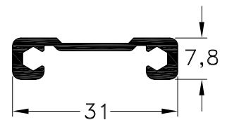
1090946 - Barra Toallera Peso: 0,24 Kg/m. Largo Std.: 6.030 mm.
