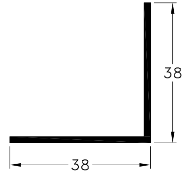
1090757 - Perfil Angulo Peso: 0,34 Kg/m. Largo Std.: 6.030 mm.
