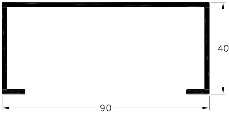
1090114 - Canal Liso 90 x 40 mm. Peso: 0,98 Kg/m. Largo Std.: 6.030 mm.
