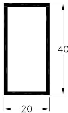
1090805 - Tubo 40 x 20 mm. Peso: 0,46 Kg/m. Largo Std.: 6.030 mm.
