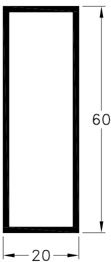
1090812 - Tubo 60 x 20 mm. Peso: 0,63 Kg/m. Largo Std.: 6.030 mm.
