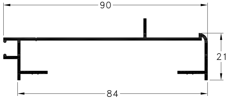
1090355 - Marco Aireador Aletado con Mosquitero Peso: 0,55 Kg/m. Largo Std.: 6.030 mm.
