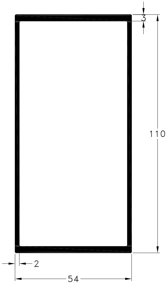
1090970 - Tubo 110 x 54 mm. Peso: 2,00 Kg/m. Largo Std.: 6.030 mm.
