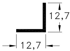
1090751 - Perfil Angulo Peso: 0,08 Kg/m. Largo Std.: 6.030 mm.
