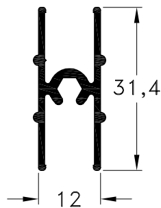
1090044 - Travesaño de Hoja Peso: 0,31 Kg/m. Largo Std.: 6.020 mm.
