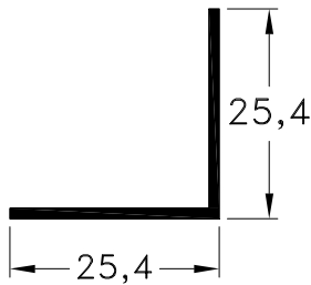
1090755 - Perfil Angulo Peso: 0,16 Kg/m. Largo Std.: 6.030 mm.
