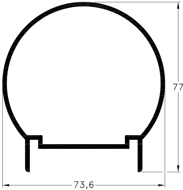
1090475 - Pasamanos Peso: 1,30 Kg/m. Largo Std.: 6.030 mm.
