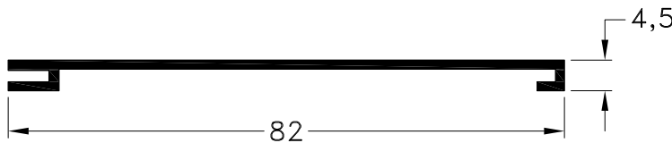
1090498 - Tapa Zócalo Peso: 0,34 Kg/m. Largo Std.: 6.030 mm.
