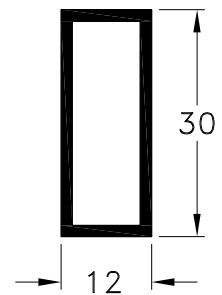
1090810 - Tubo 30 x 12 mm. Peso: 0,32 Kg/m. Largo Std.: 6.030 mm.
