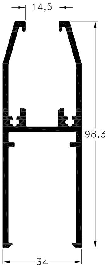
1090110 - Zócalo Peso: 1,66 Kg/m. Largo Std.: 6.030 mm.
