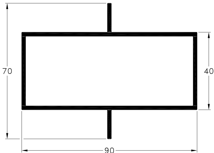
1090117 - Tubo con Dos Alas 90 x 40 mm. Peso: 1,52 Kg/m. Largo Std.: 6.030 mm.
