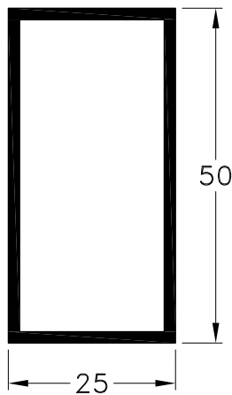
1090809 - Tubo 50 x 25 mm. Peso: 0,55 Kg/m. Largo Std.: 6.030 mm.
