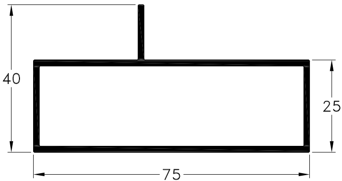
1090112 - Tubo con Un Ala 75 x 25 mm. Peso: 0,90 Kg/m. Largo Std.: 6.030 mm.
