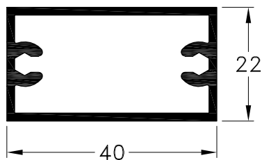
1090476 - Parante Peso: 0,61 Kg/m. Largo Std.: 6.030 mm.
