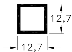
1090587 - Tubo 12,7 x 12,7 mm. Peso: 0,15 Kg/m. Largo Std.: 6.020 mm.
