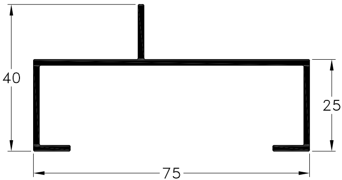
1090119 - Canal con Un Ala 75 x 25 mm. Peso: 0,66 Kg/m. Largo Std.: 6.030 mm.
