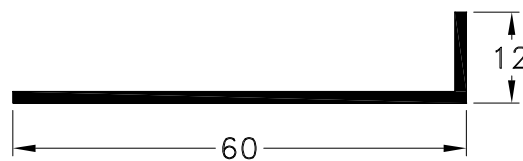
1090125 - Perfil Angulo Peso: 0,29 Kg/m. Largo Std.: 6.030 mm.
