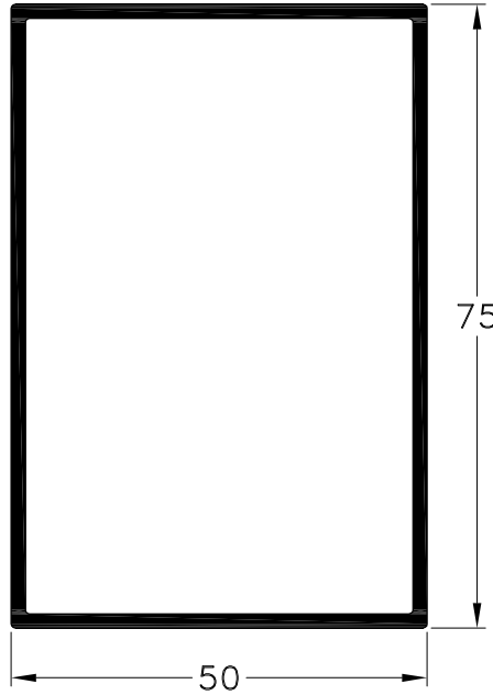
1090464 - Tubo 75 x 50 mm. Peso: 1,12 Kg/m. Largo Std.: 6.030 mm.
