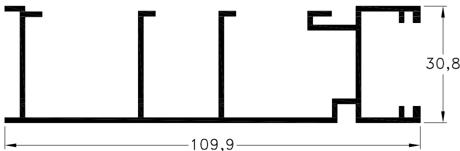
1090499 - Zócalo Peso: 1,04 Kg/m. Largo Std.: 6.030 mm.
