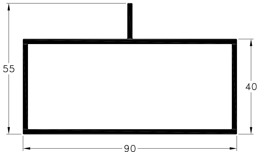
1090116 - Tubo con Un Ala 90 x 40 mm. Peso: 1,44 Kg/m. Largo Std.: 6.030 mm.
