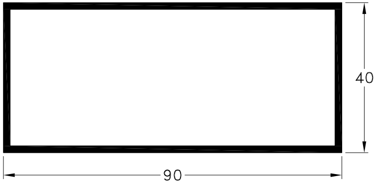
1090458 - Tubo 90 x 40 mm. Peso: 1,23 Kg/m. Largo Std.: 6.030 mm.
