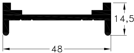
1090477 - Base de Pasamanos Peso: 0,56 Kg/m. Largo Std.: 6.030 mm.
