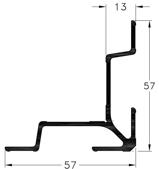
1090063 - Escuadra Universal Pesada Peso: 0,74 Kg/m. Largo Std.: 6.030 mm.
