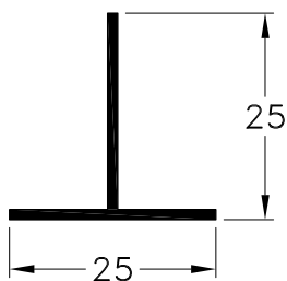
1090830 - Perfil T Peso: 0,16 Kg/m. Largo Std.: 6.030 mm.
