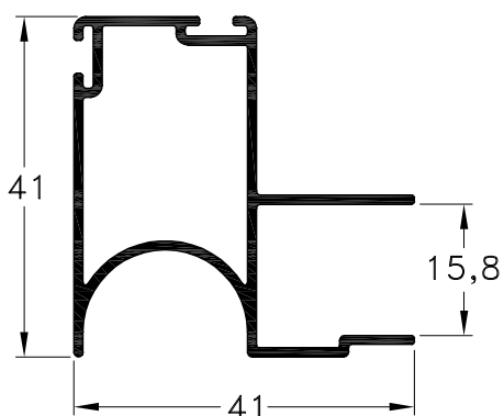
1090155 - Parante de 15 mm. Peso: 0,53 Kg/m. Largo Std.: 5.200 mm.
