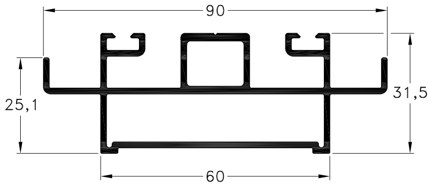
1090192 - Travesaño Peso: 1,27 Kg/m. Largo Std.: 6.030 mm.
